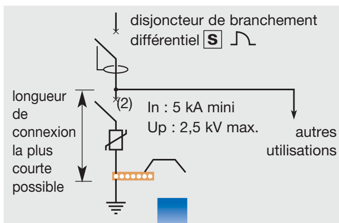
Réduire au maximum la longueur des connexions
