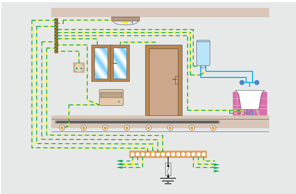
Liaison équipotentielle locale de la salle d'eau : solution particulièrement recommandée par la norme.
