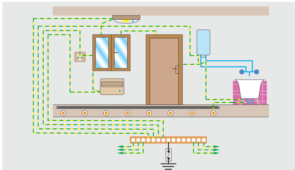
Liaison équipotentielle locale de la salle d'eau
