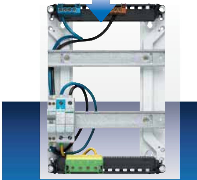
Réduire au maximum la longueur des connexions
